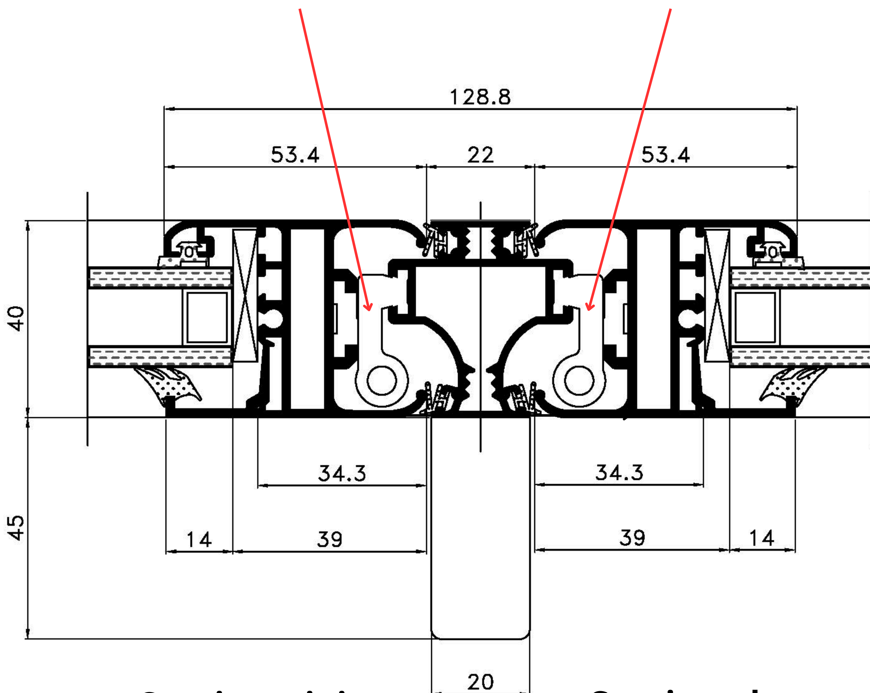
Cerniera sinistra
