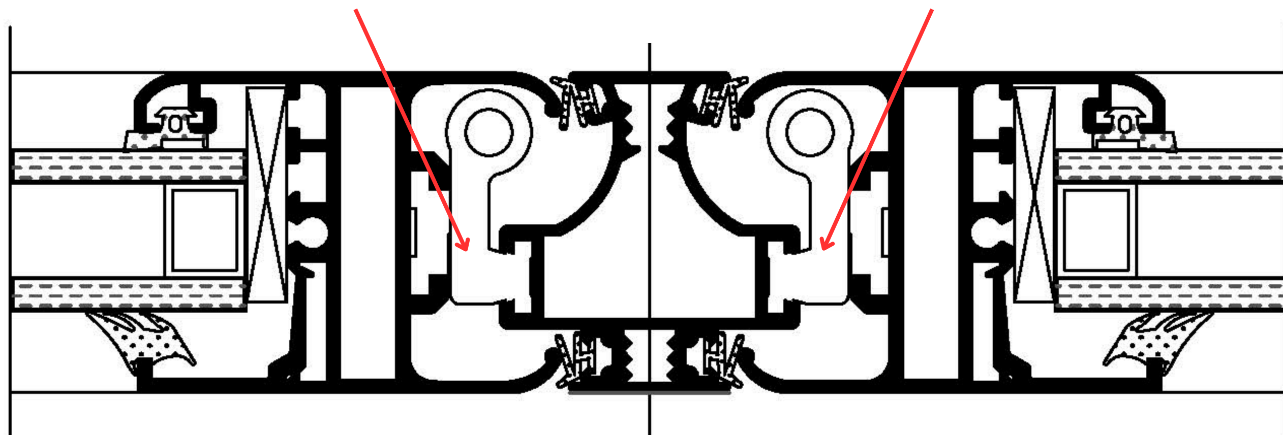
Cerniera sinistra
